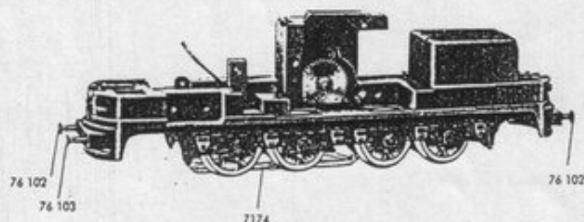
Fig. 3 Treibgestell
