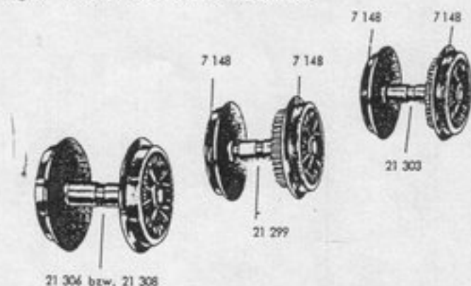
Fig. 5 Treibradsätze und Radsätze
