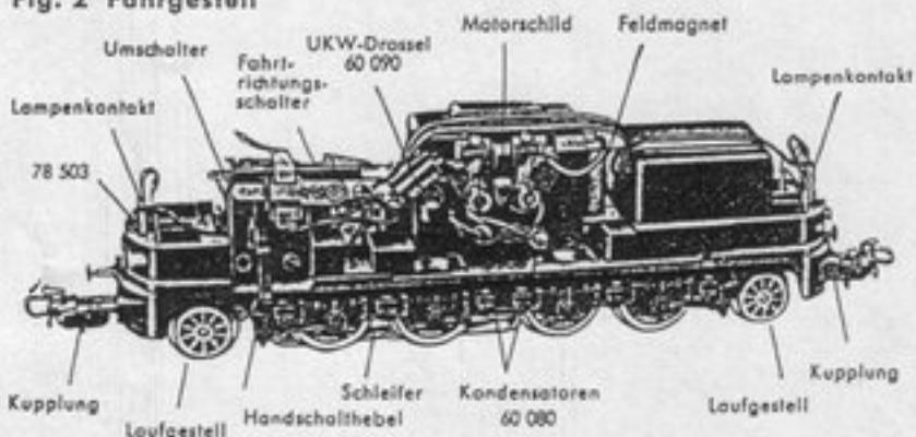
Fig. 2 Fahrgestell
