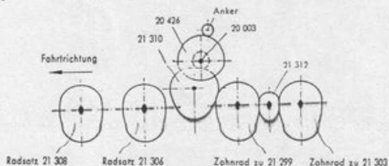
Fig. 4 Anordnung der Getrieberäder
